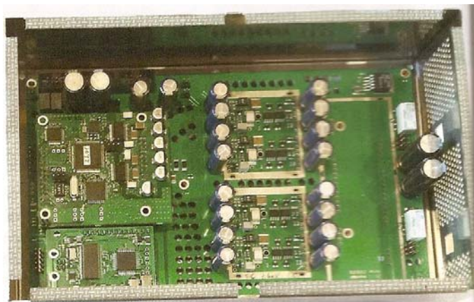
Der DAC im Purist Statement 7 bietet Upsampling ohne Interpolationsfilter und weist auch keine analogen Filter auf. Der Hersteller bescheinigt der Schaltung enorme Bandbreite bis über 100 Kilohertz.
